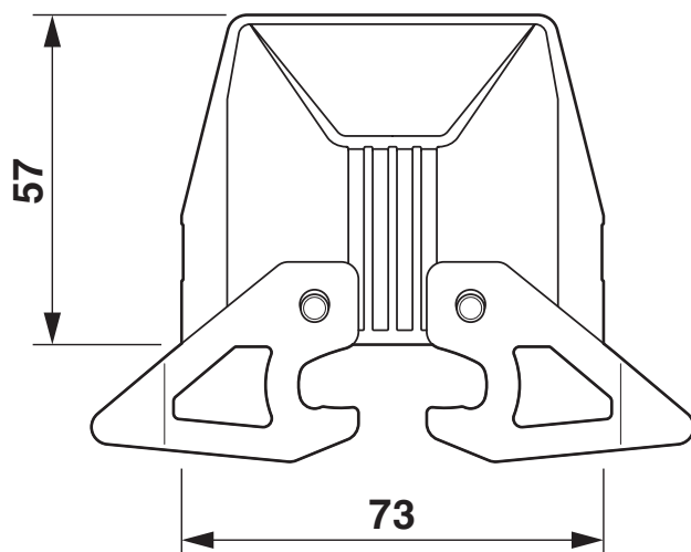
Rysunek wymiarowy
