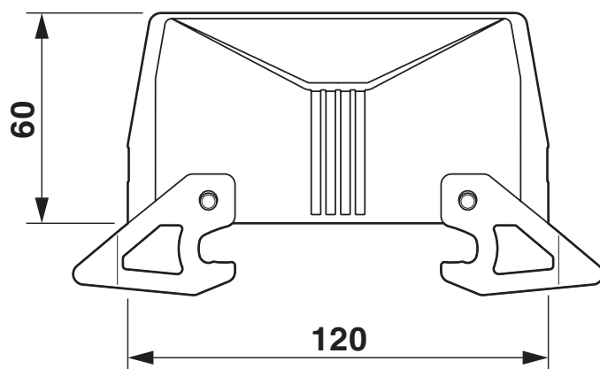
Rysunek wymiarowy
