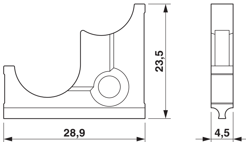
Rysunek wymiarowy
