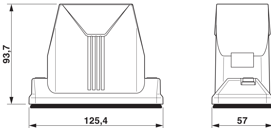
Rysunek wymiarowy
