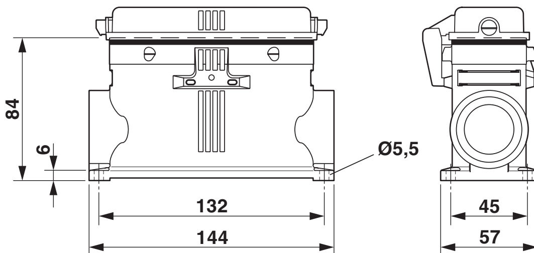
Rysunek wymiarowy
