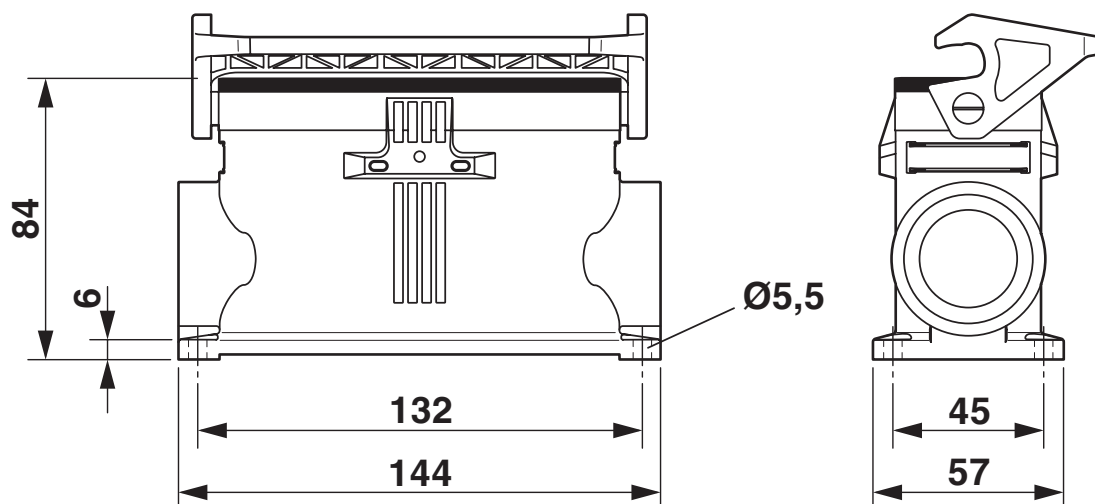
Rysunek wymiarowy
