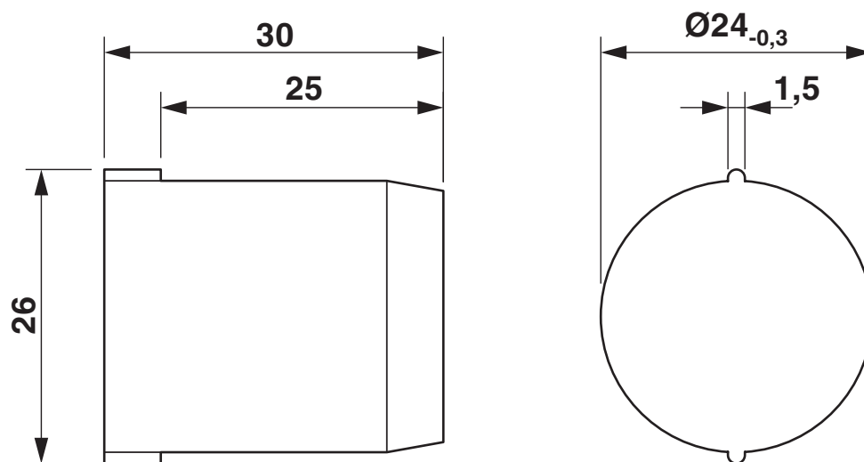
Rysunek wymiarowy
