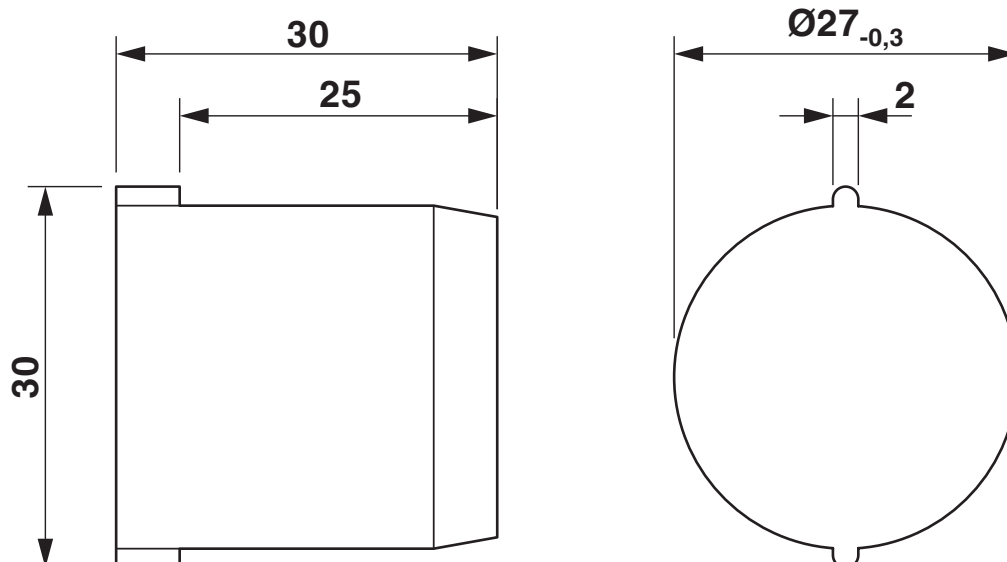
Rysunek wymiarowy
