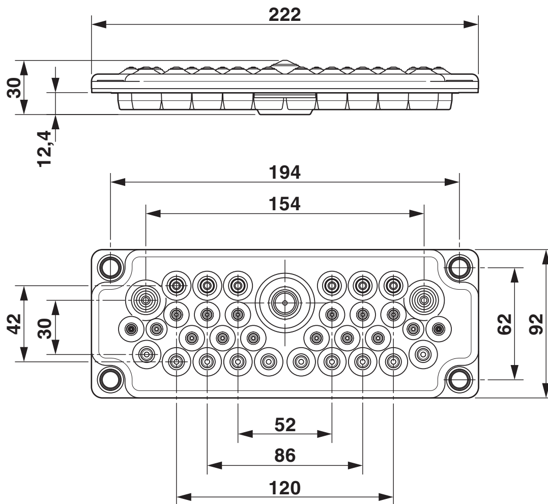
Rysunek wymiarowy
