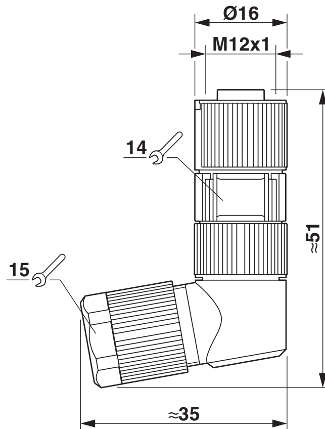
Rysunek wymiarowy
