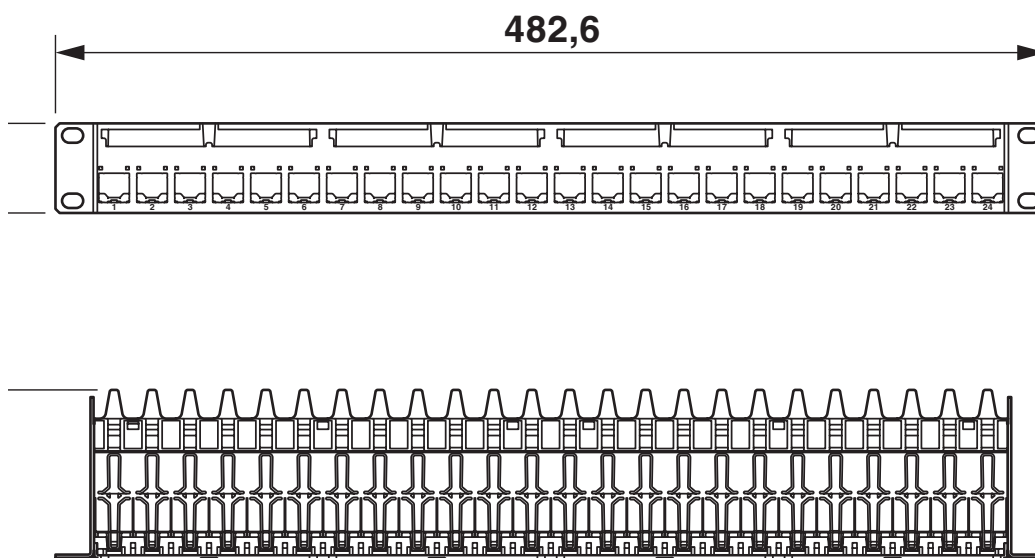
Rysunek wymiarowy
