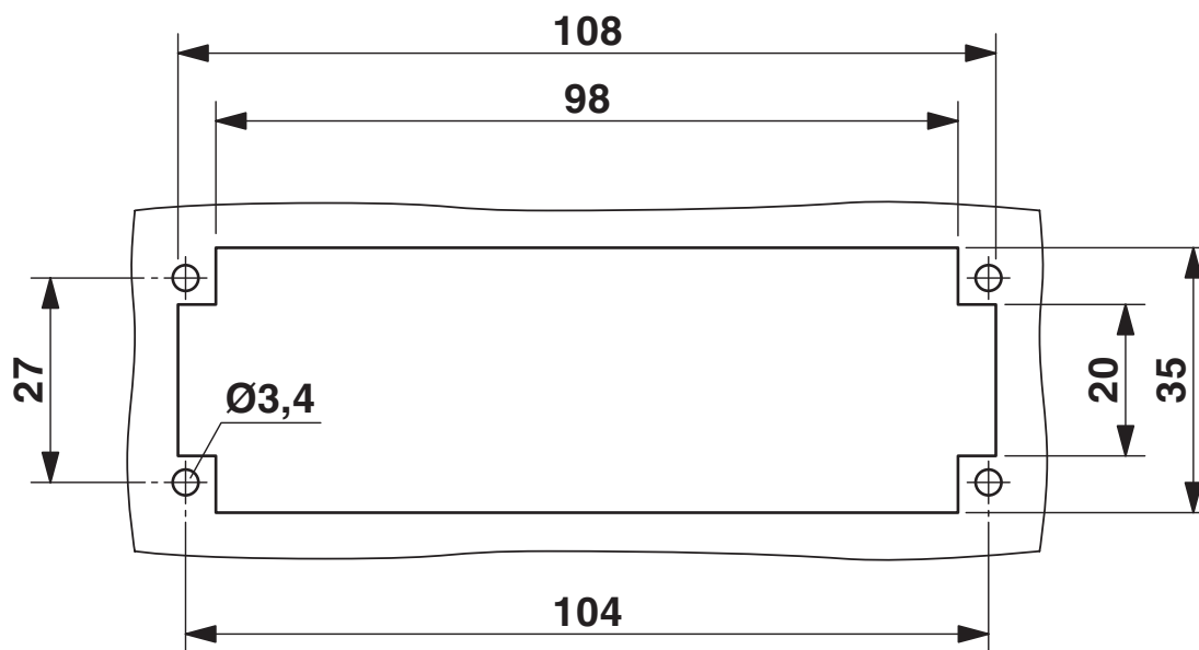
Wycięcie montażowe przy zastosowaniu bez obudowy
