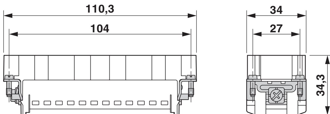
Wkładka styków męskich
