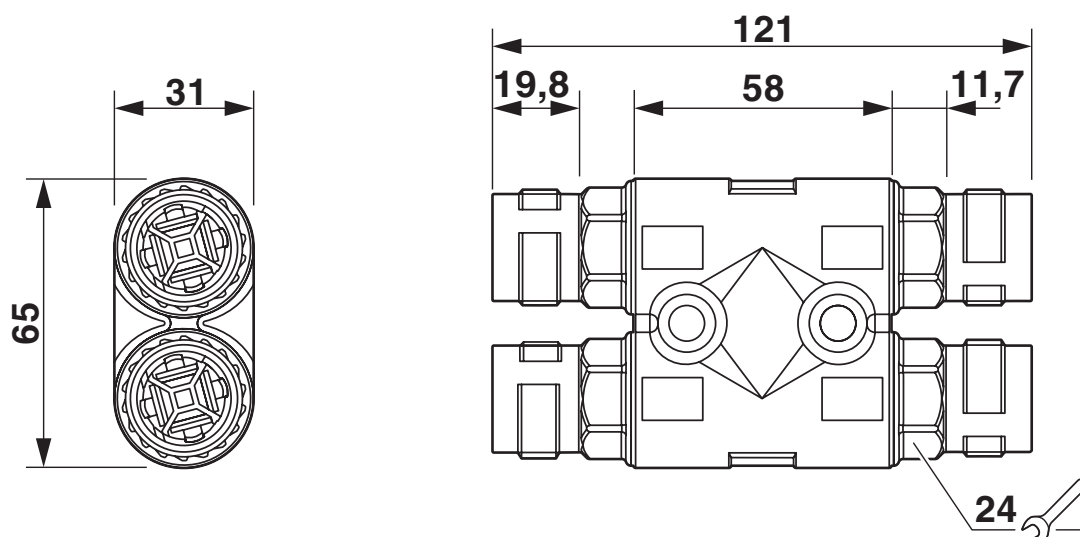
Rysunek wymiarowy
