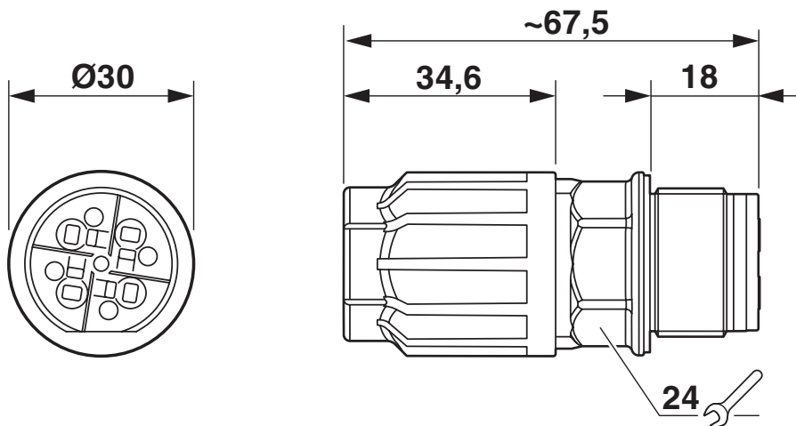
Rysunek wymiarowy
