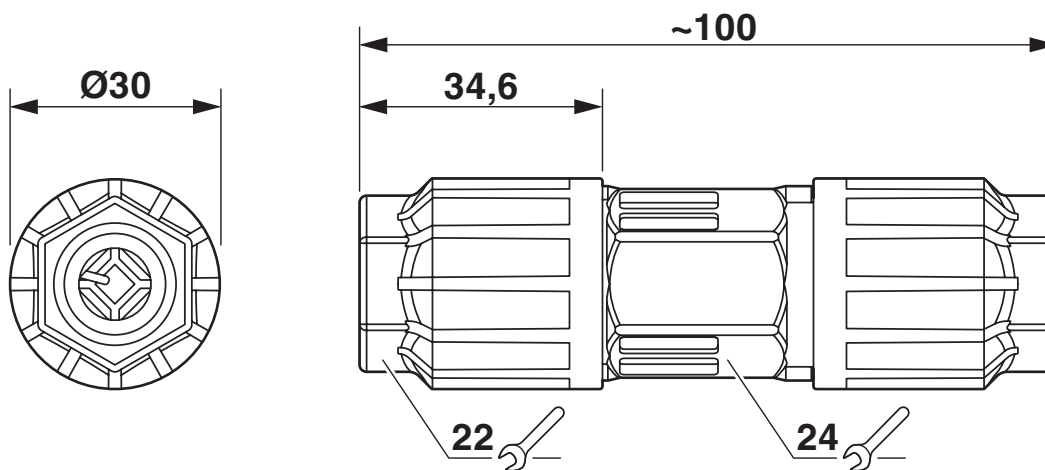
Rysunek wymiarowy
