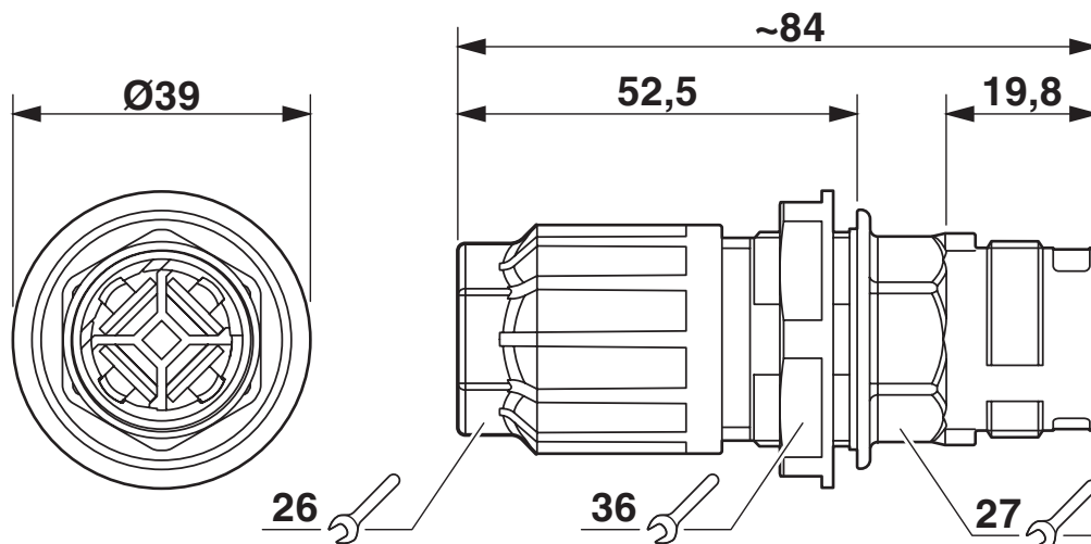
Rysunek wymiarowy
