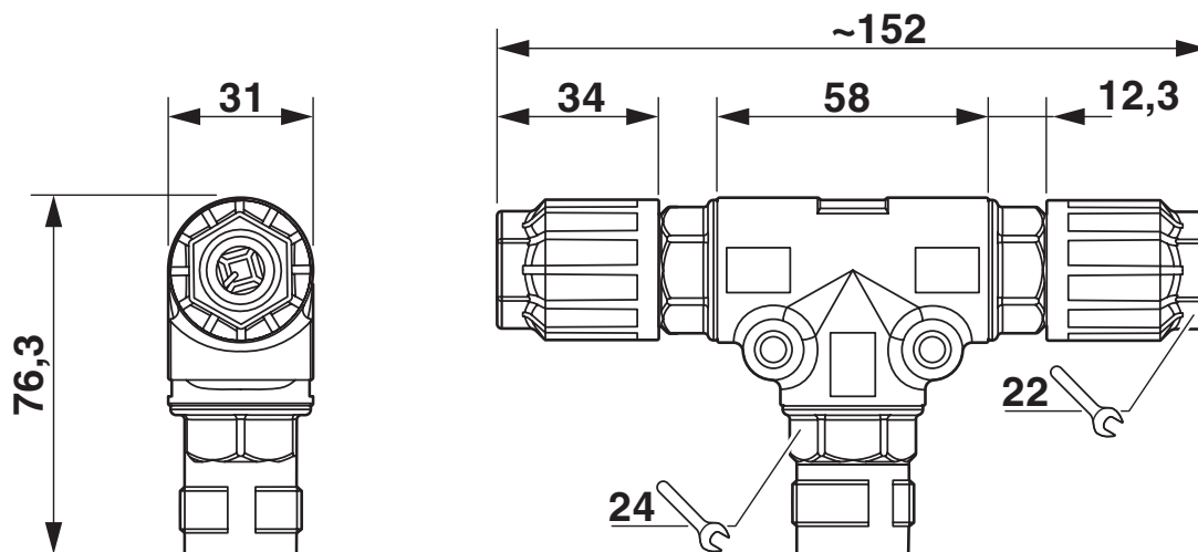
Rysunek wymiarowy
