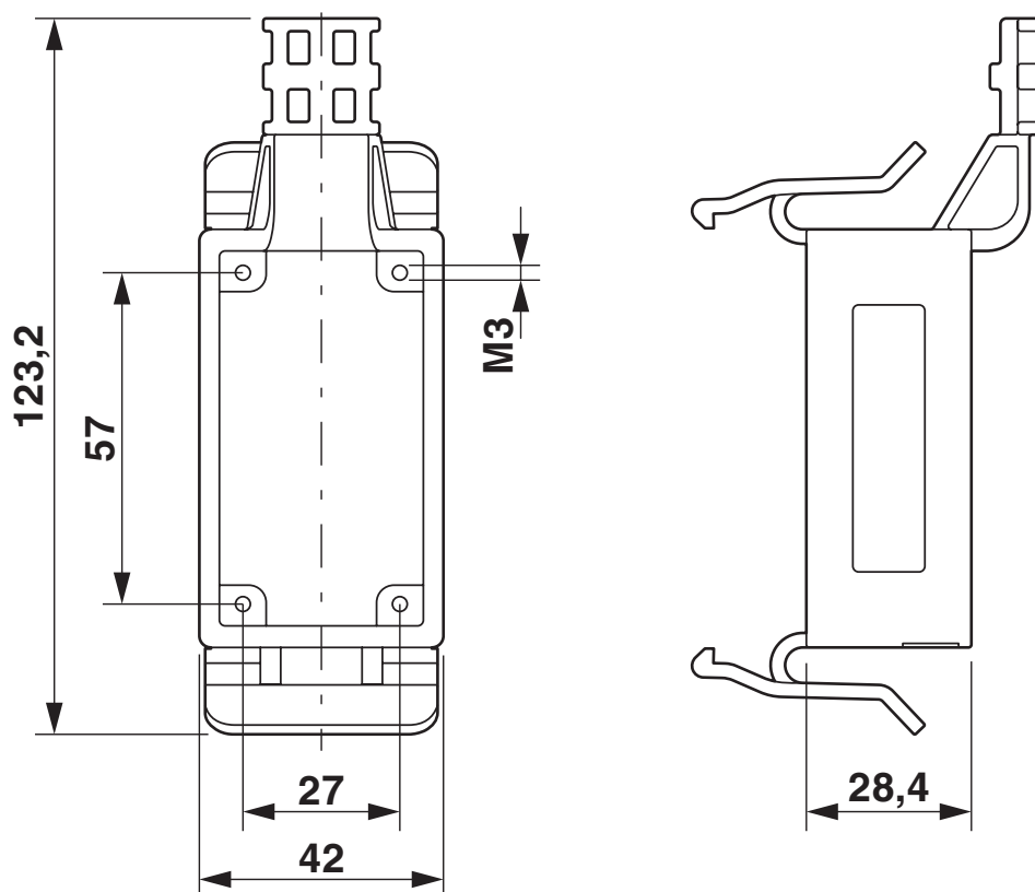
Rysunek wymiarowy
