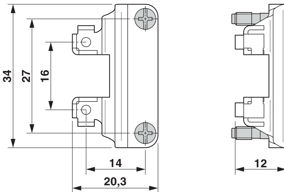
Rysunek wymiarowy
