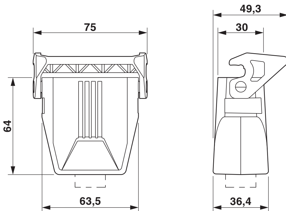
Rysunek wymiarowy
