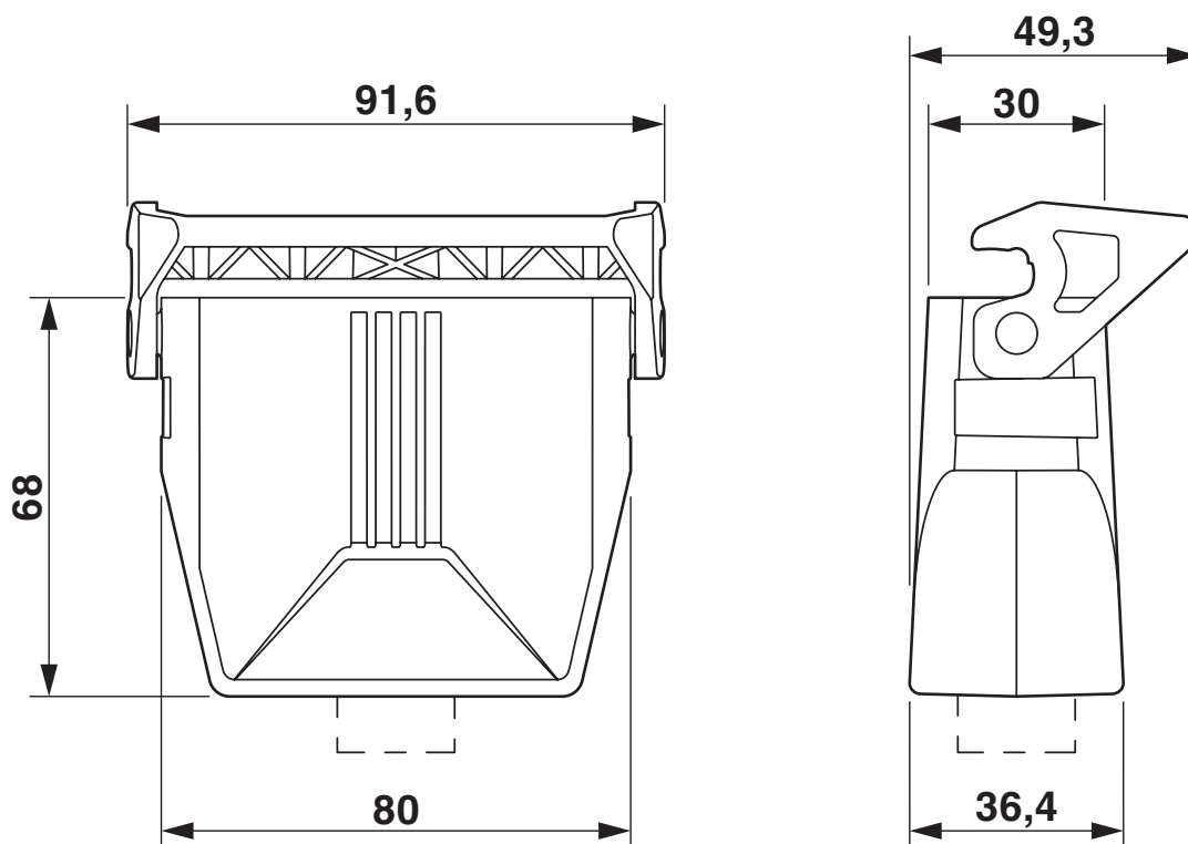
Rysunek wymiarowy
