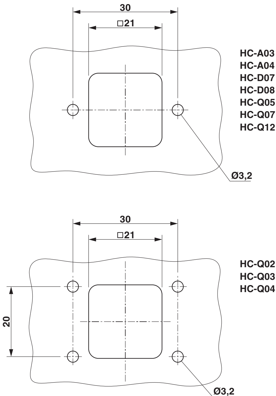
Rysunek wymiarowy
