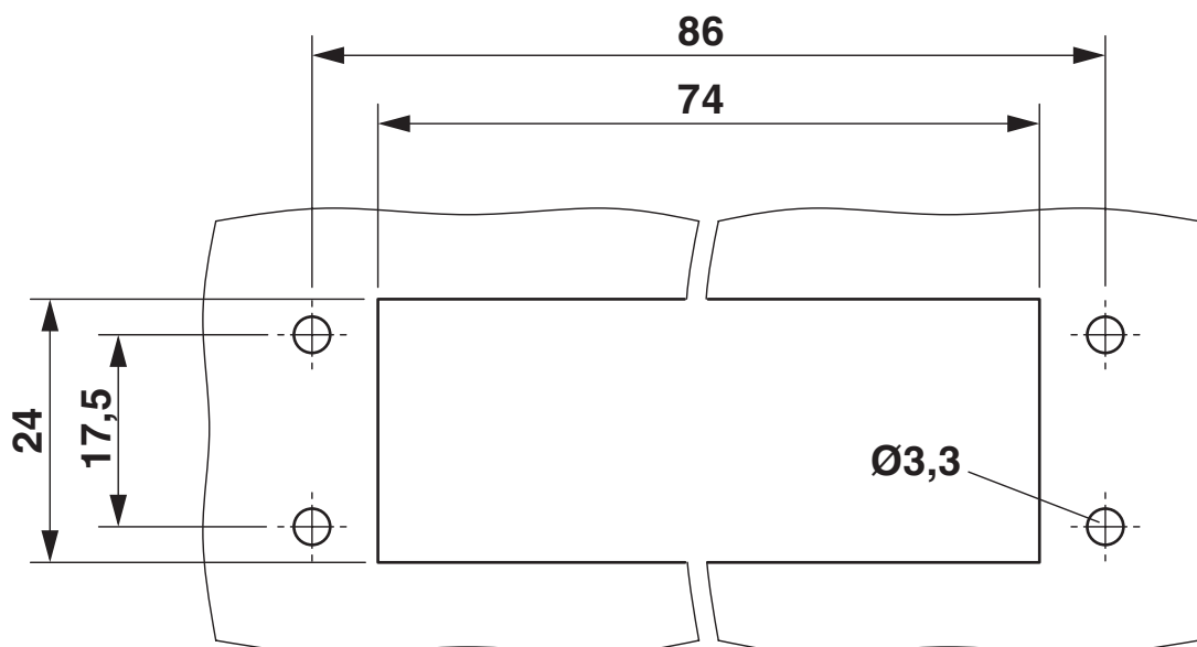
Rysunek wymiarowy
