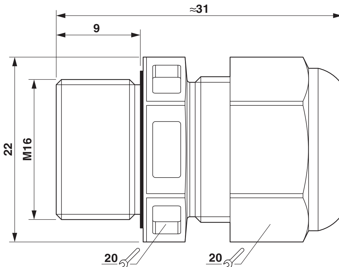
Rysunek wymiarowy
