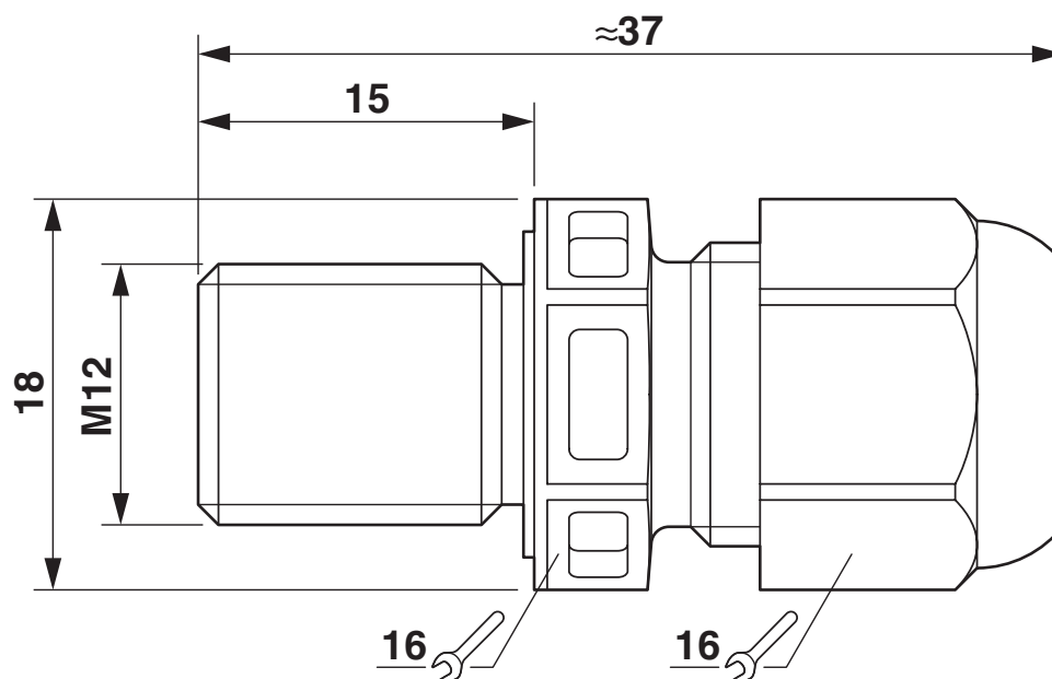
Rysunek wymiarowy
