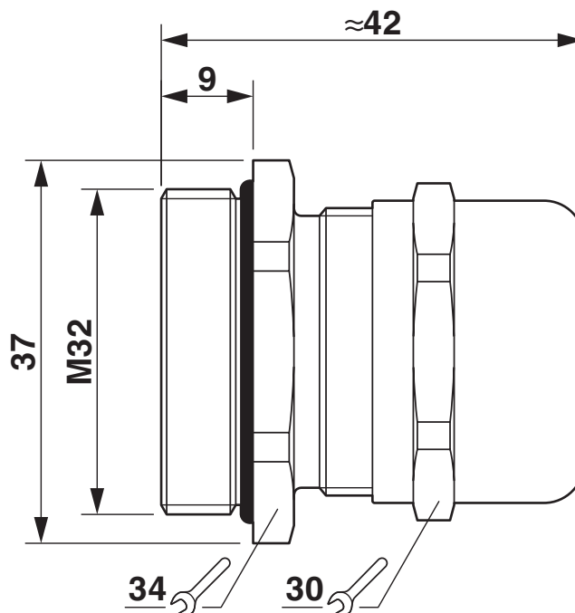
Rysunek wymiarowy
