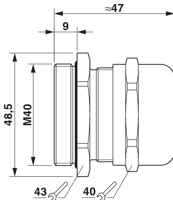
Rysunek wymiarowy
