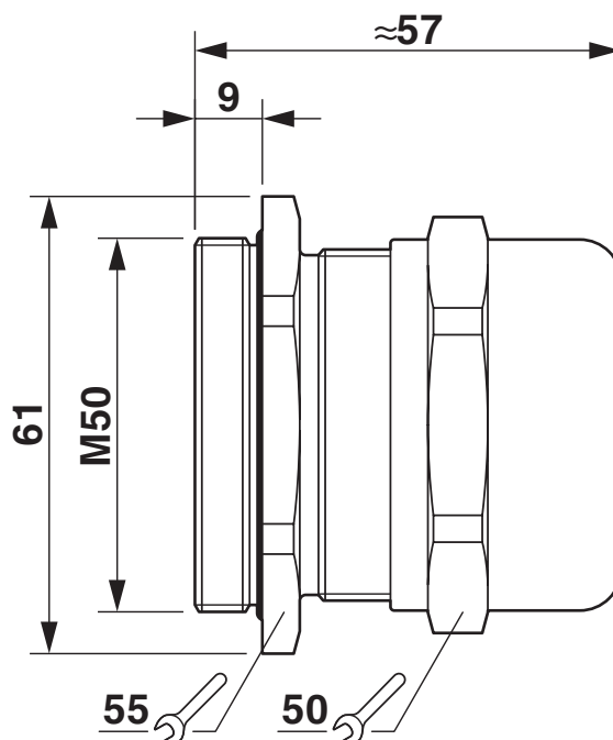
Rysunek wymiarowy
