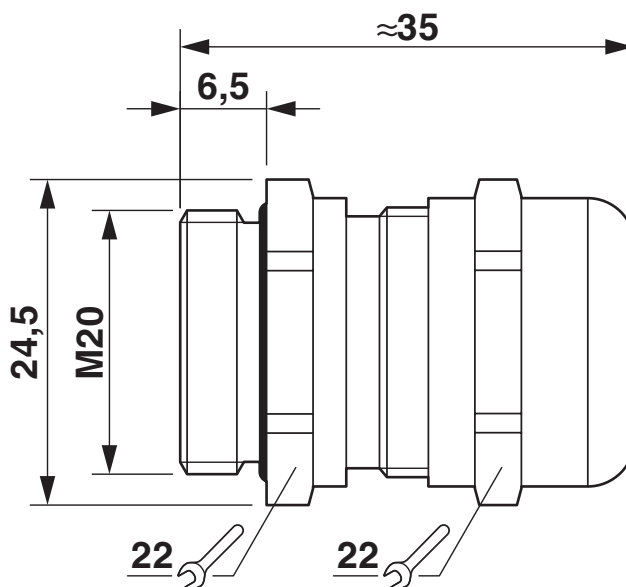
Rysunek wymiarowy
