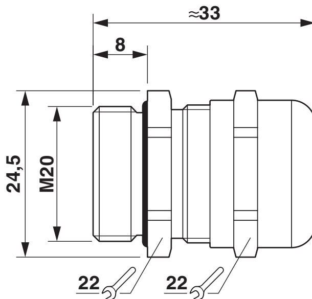
Rysunek wymiarowy
