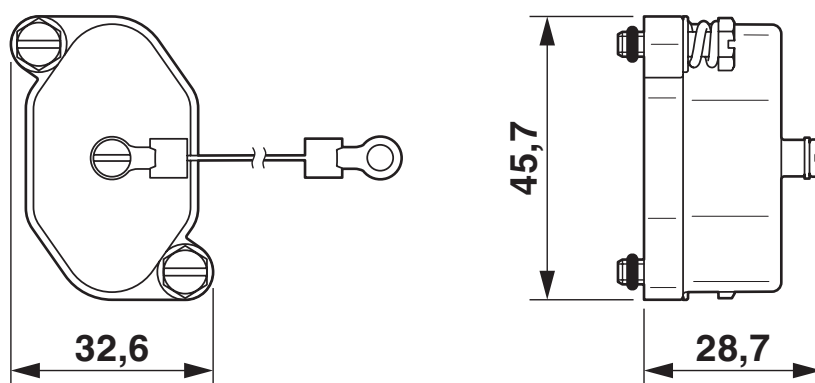
Rysunek wymiarowy
