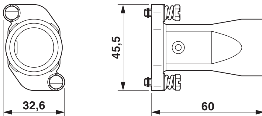
Rysunek wymiarowy
