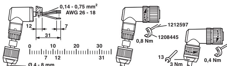
rysunek funkcyjny
