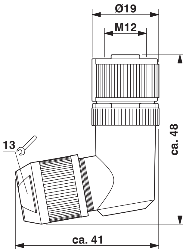
Rysunek wymiarowy
