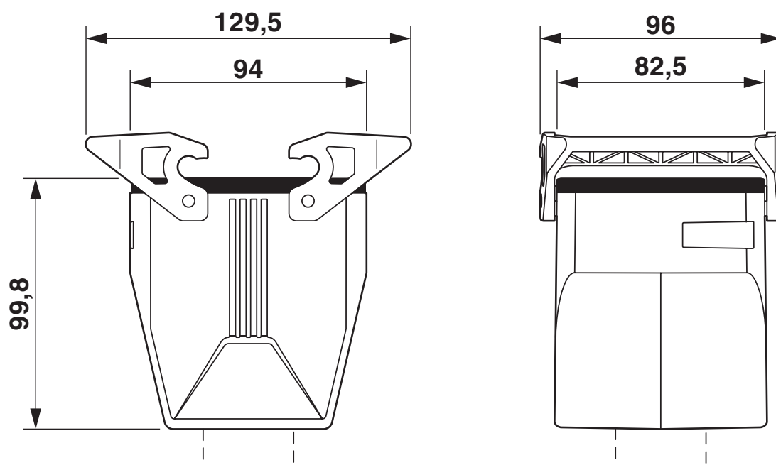
Rysunek wymiarowy
