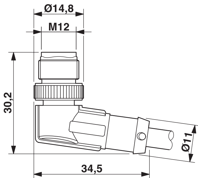
Rysunek wymiarowy
