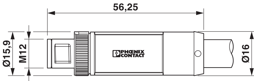
Wtyk męski M12 x 1, prosty, ekranowany
