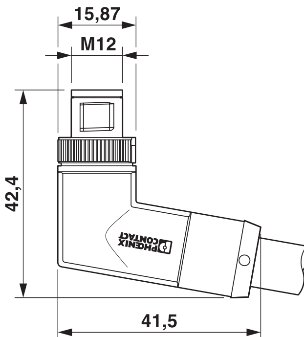
Rysunek wymiarowy
