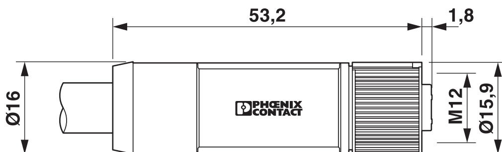
Rysunek wymiarowy
