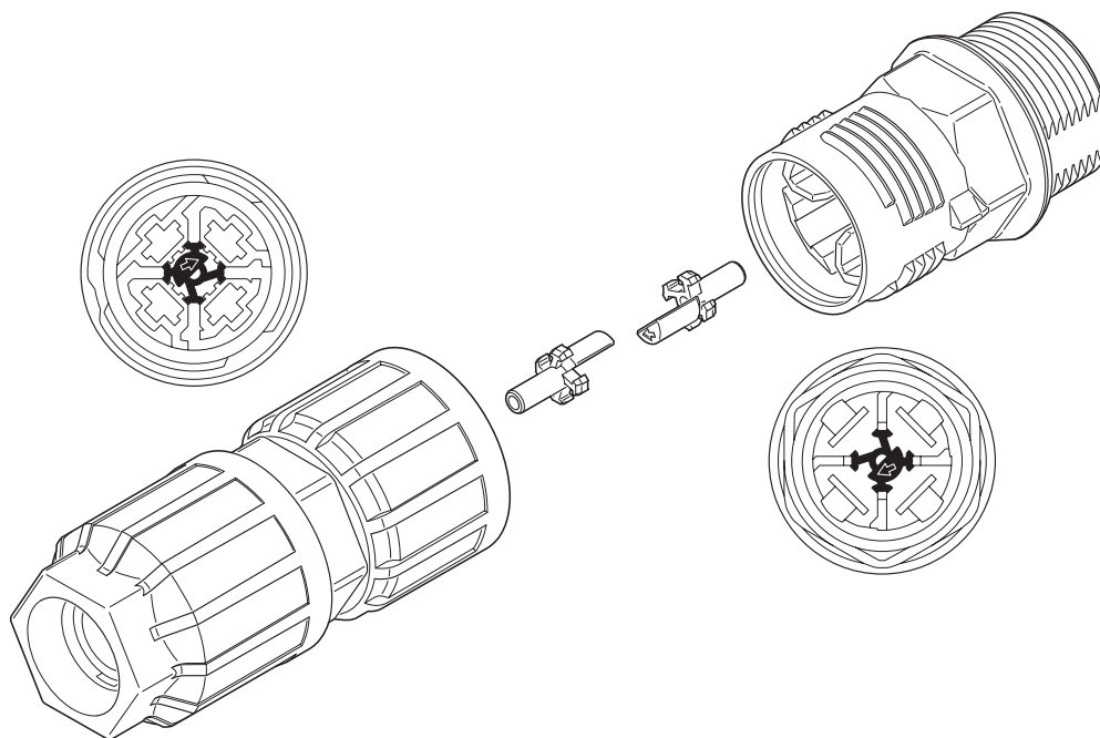
Rysunek schematyczny
