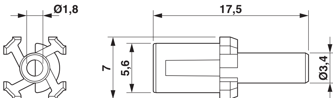
Rysunek wymiarowy
