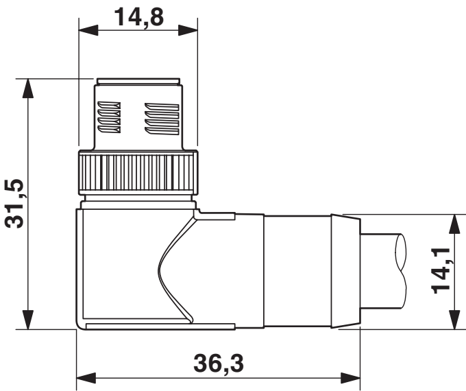
Rysunek wymiarowy
