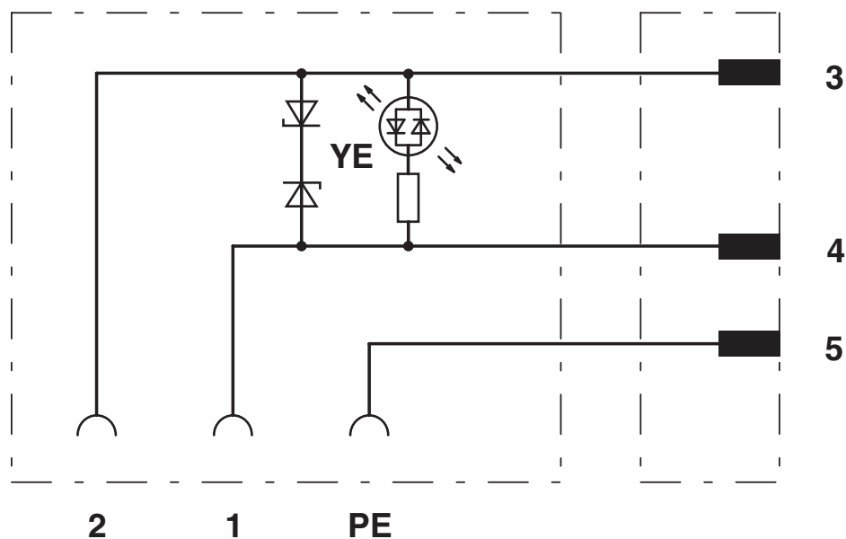
Schemat
