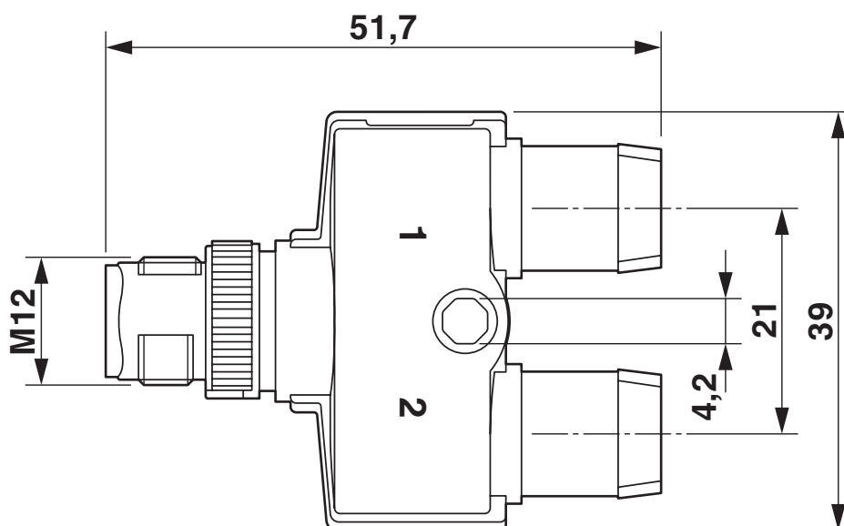
Rysunek wymiarowy
