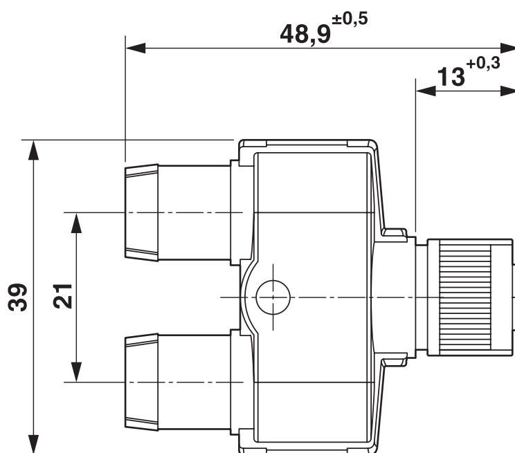
Rysunek wymiarowy
