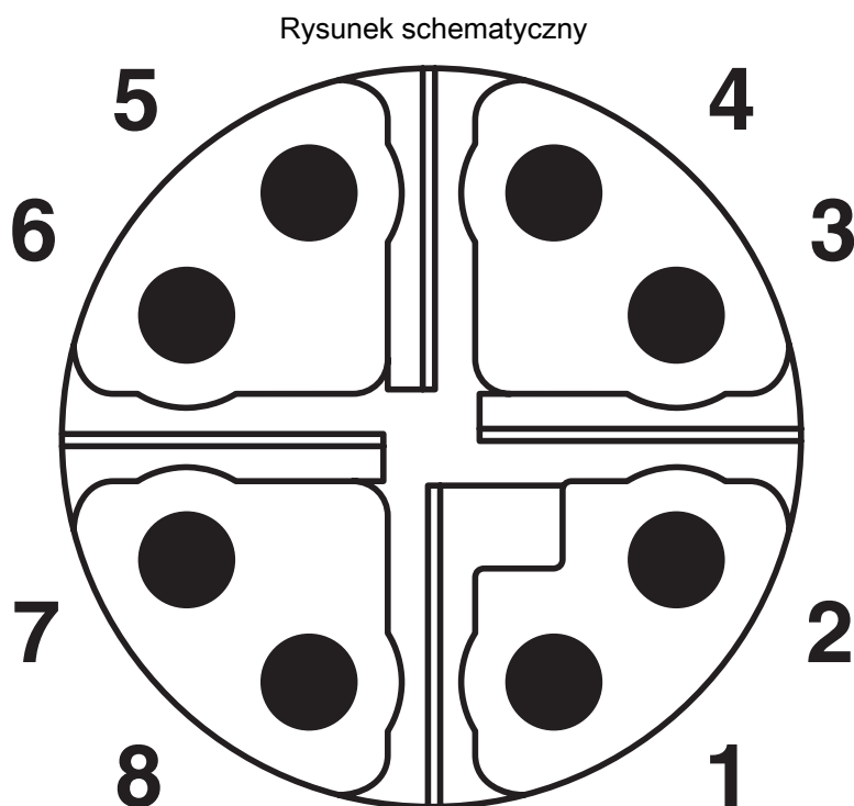
Układ styków, wtyk M12 CAT6 A , 8-biegunowy, widok od strony wtyku
