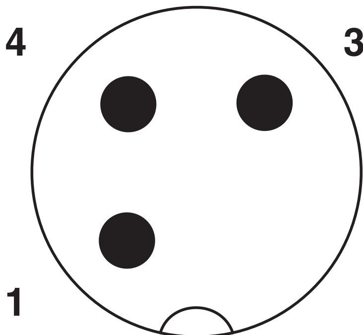
Układ biegunów wtyku męskiego M12, 3-biegunowy, z kodowaniem typu A, widok od strony z kołkami
