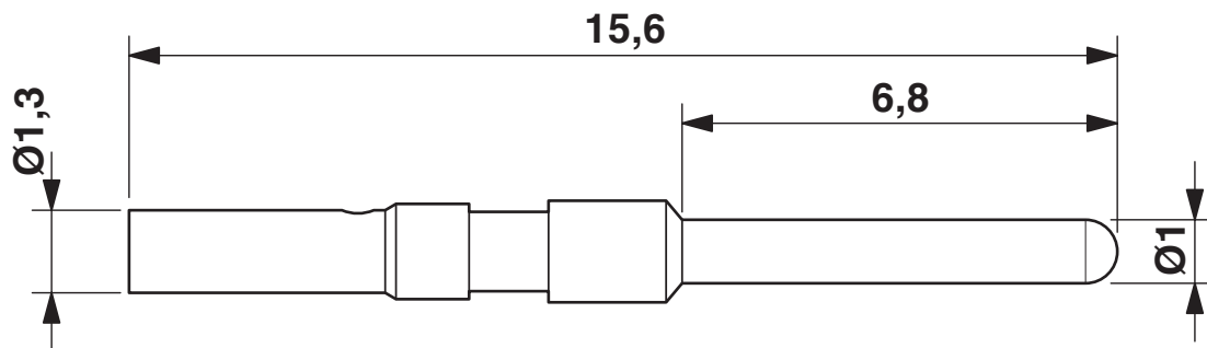
Rysunek wymiarowy
