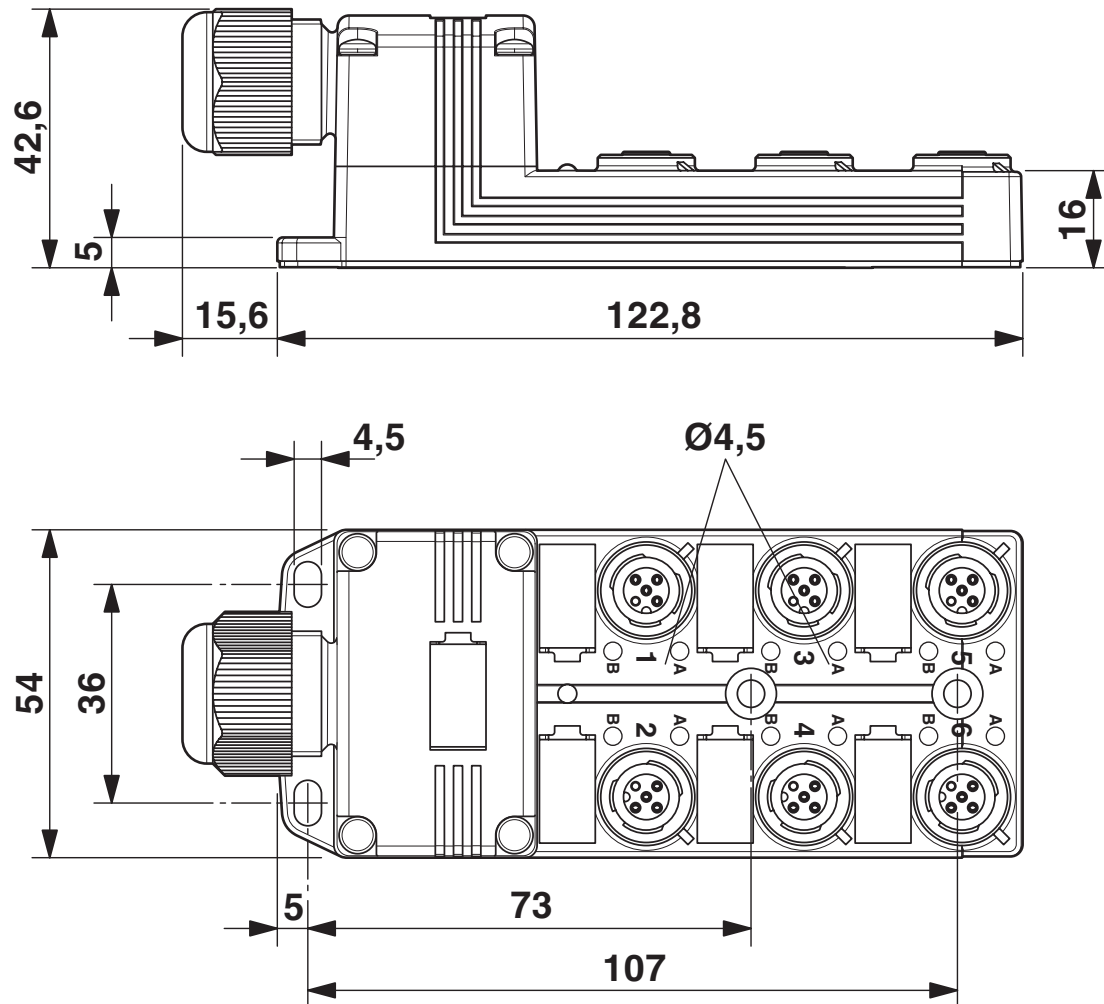
Rysunek wymiarowy
