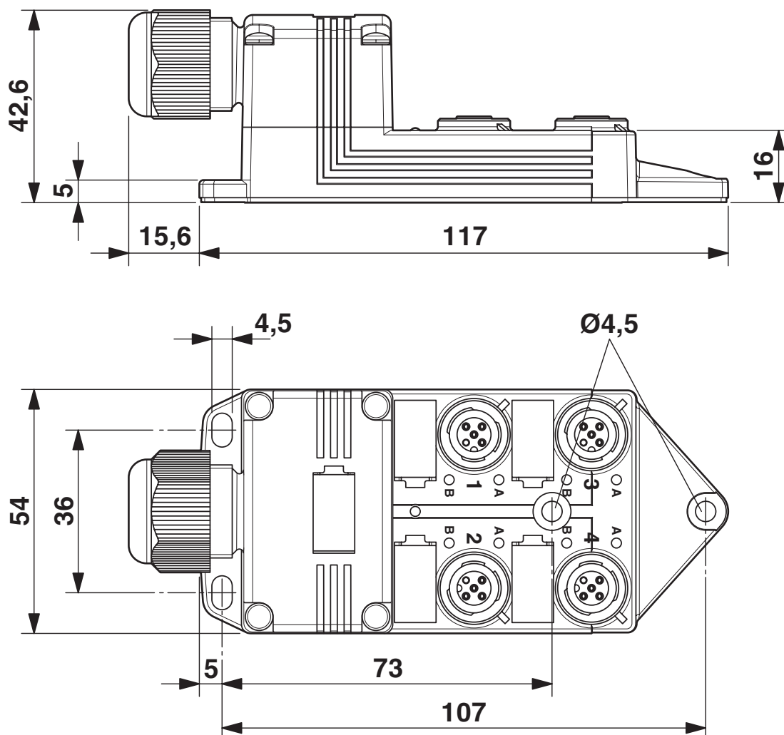
Rysunek wymiarowy
