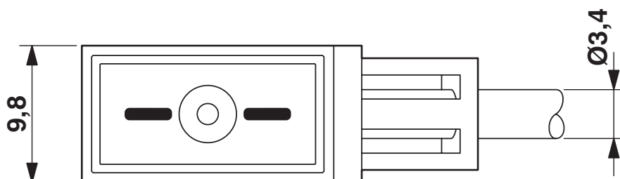
Rysunek wymiarowy
