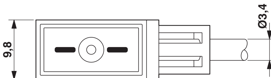
Rysunek wymiarowy
